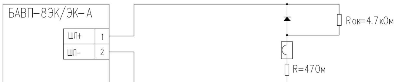
Подключение световых извещателей к БАКП-8ЭК/ЭК-А Тип шлейфа "Реле с контролем цепи"
